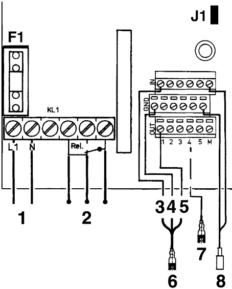
Abbildung 7: Elektrischer Anschluss OM 5+1
