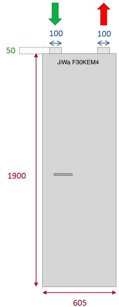
FRONT VY
